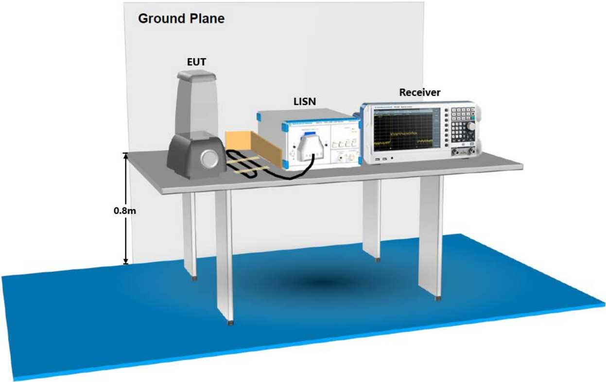
图一：EMI-CE100 基础版 EMI 诊断测试系统示例
