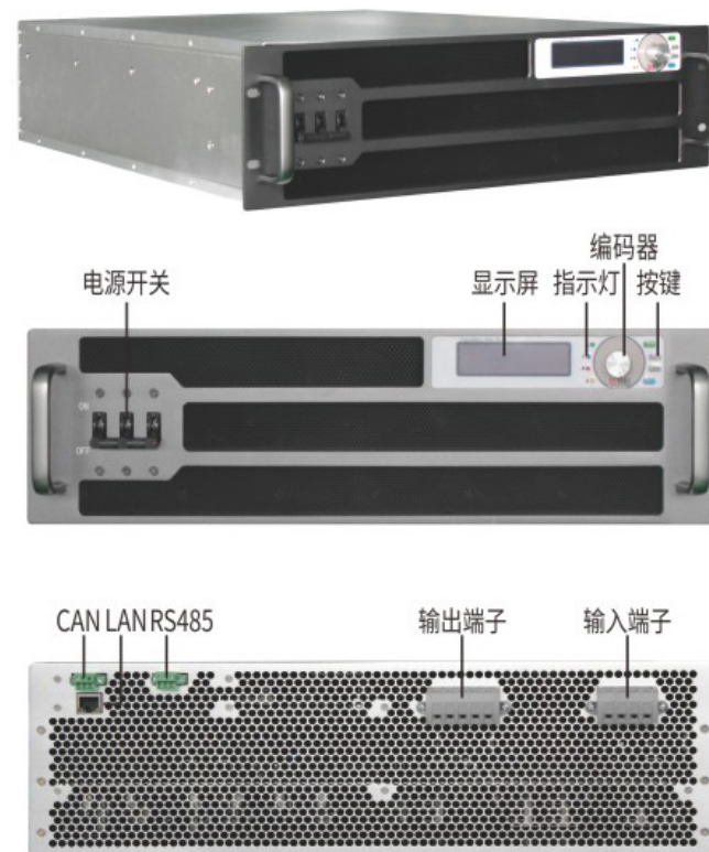
DWFP S1-3315/115E 外观图
