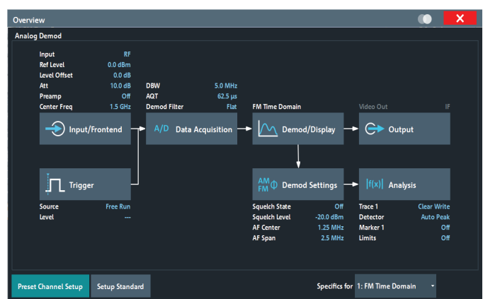
模拟解调菜单概览：可在此菜单中完成所有设置。
