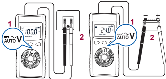
交流电压
