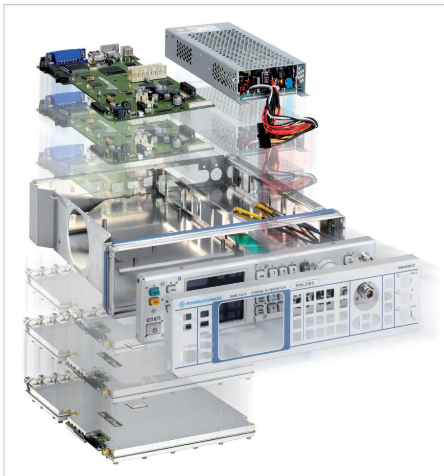
R&S®SMB100A 的各个模块都很小，意味着高可靠性和易于维护（图中为 6 GHz 型号）。
