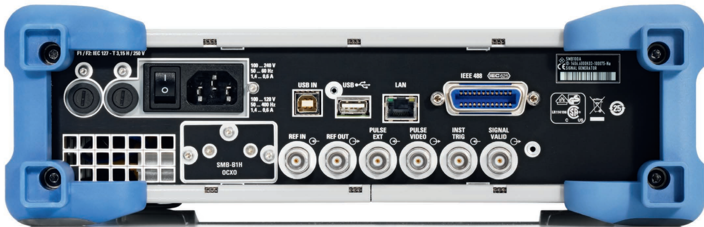
R&S®SMB100A 后视图。
