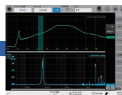
FFT 显示
