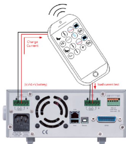
模拟充电电源和负载电流测试
