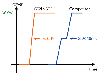
拉载功率波形图
