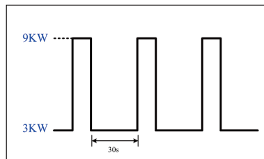
拉载波形
